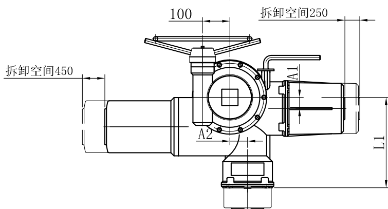
IMC100~300带BA系列外形尺寸
